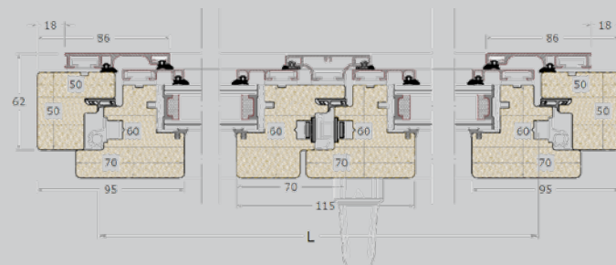
Sezione orizzontale finestra e portafinestra
