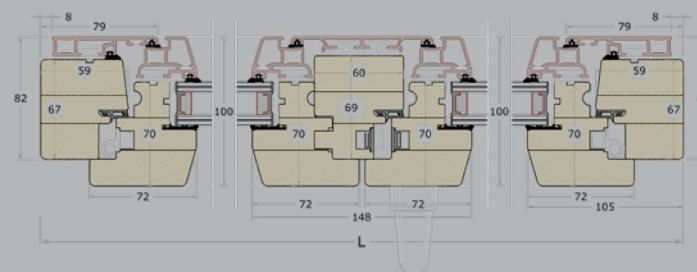
Sezione orizzontale finestra e portafinestra
