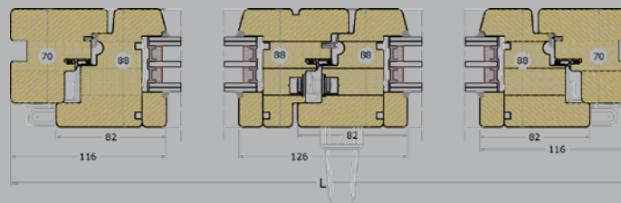
Sezione orizzontale finestra e portafinestra
