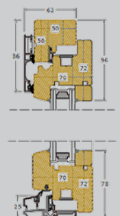
Soglia inferiore finestra e portafinestra
