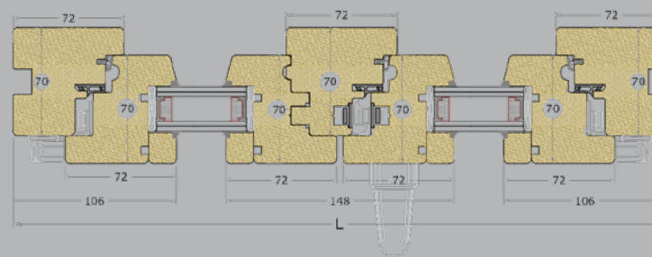
Sezione orizzontale finestra e portafinestra
